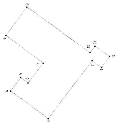
5.12. Чертеж границ земельного участка с кадастровым номером 70:22:0010104.3/11 М 1:1000
